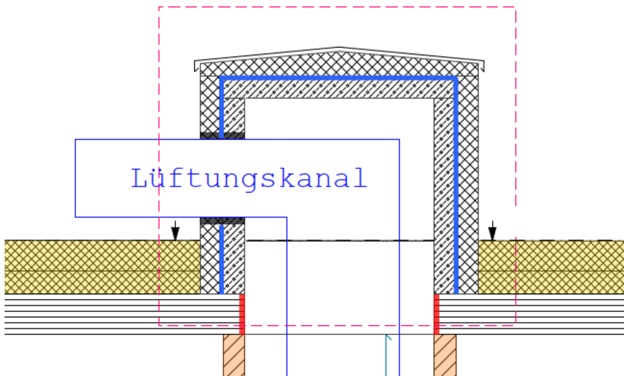
schematische Darstellung Dachdurchführung Lüftung
