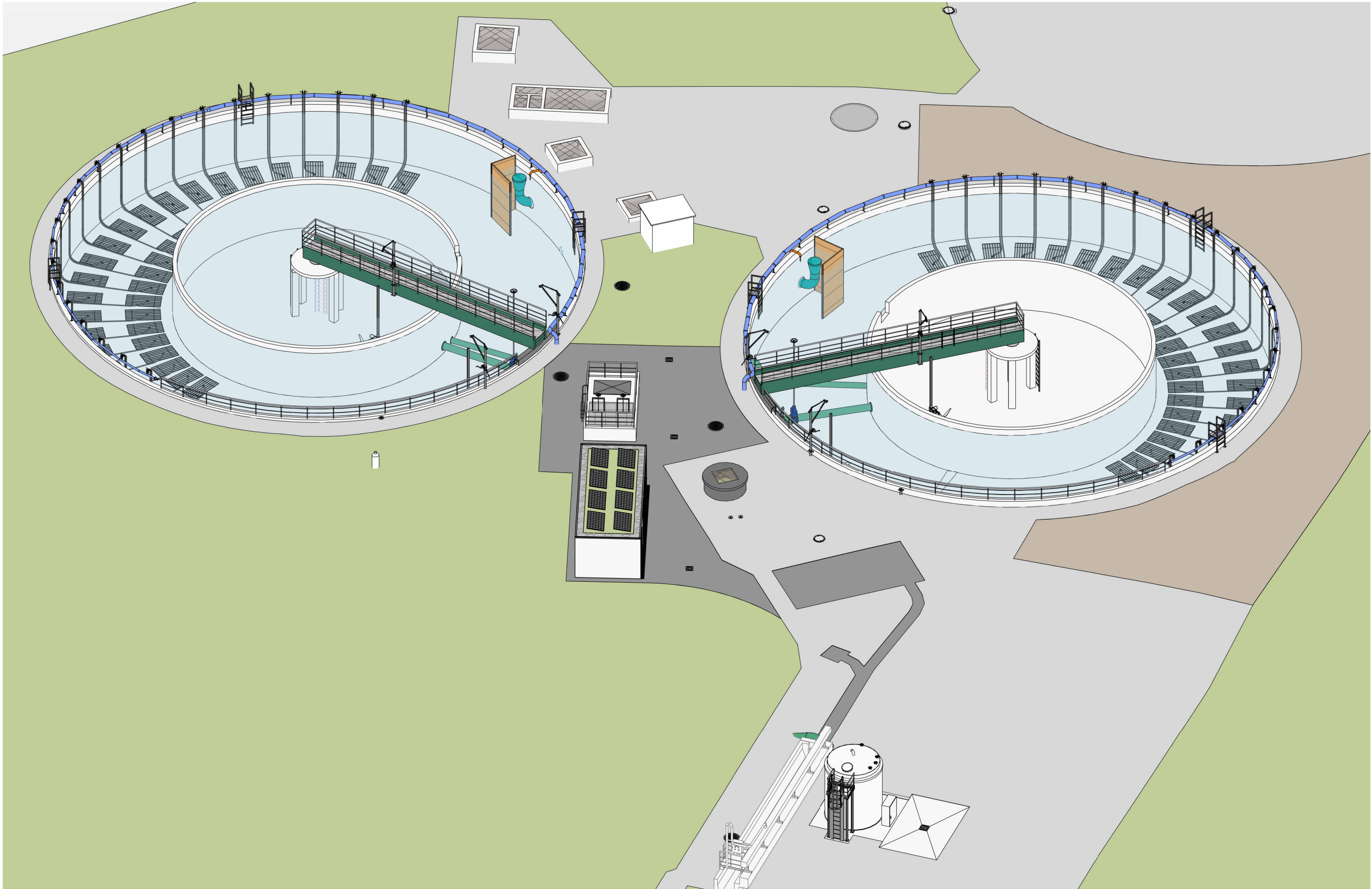
3D Ansicht
