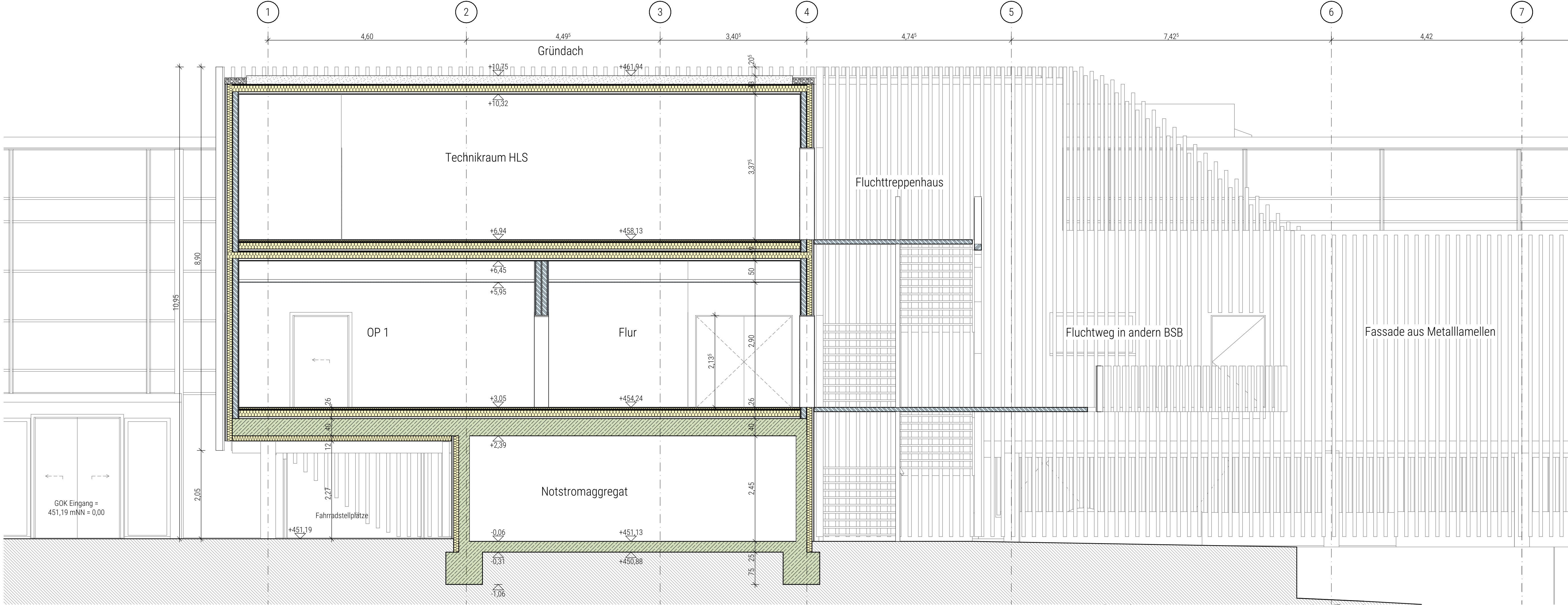
Schnitt BB 1:50
