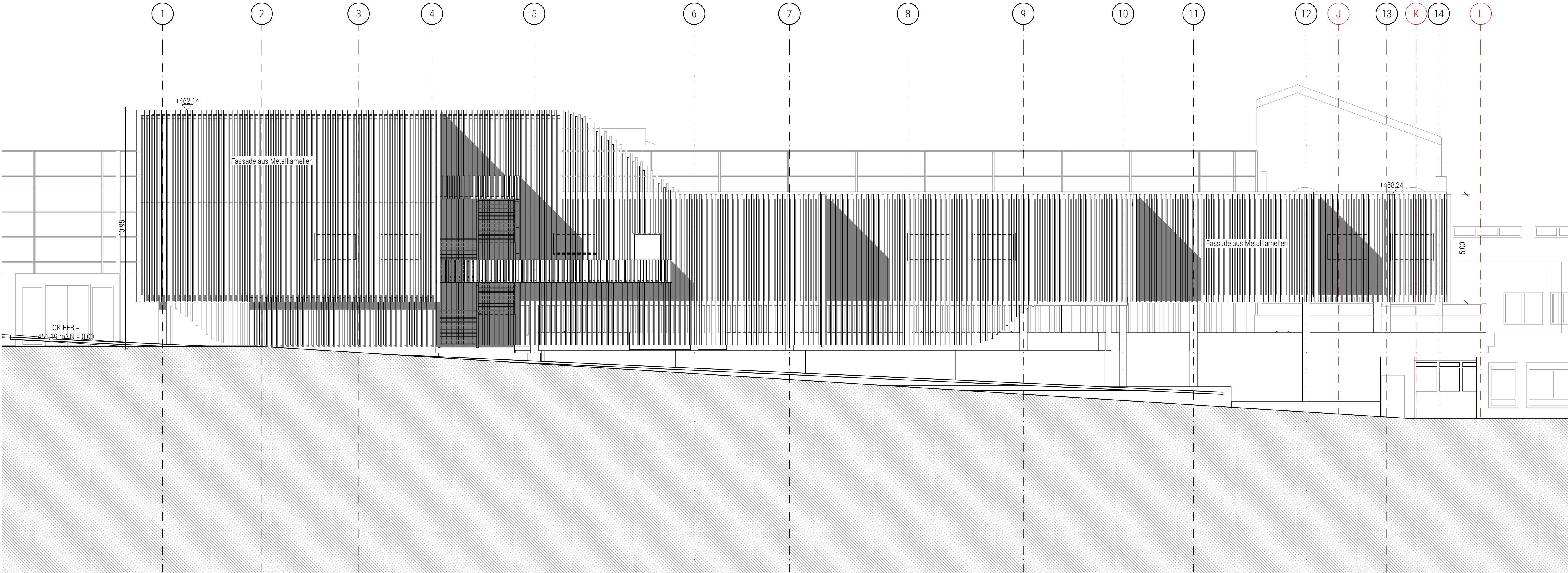
Westansicht 1:100
