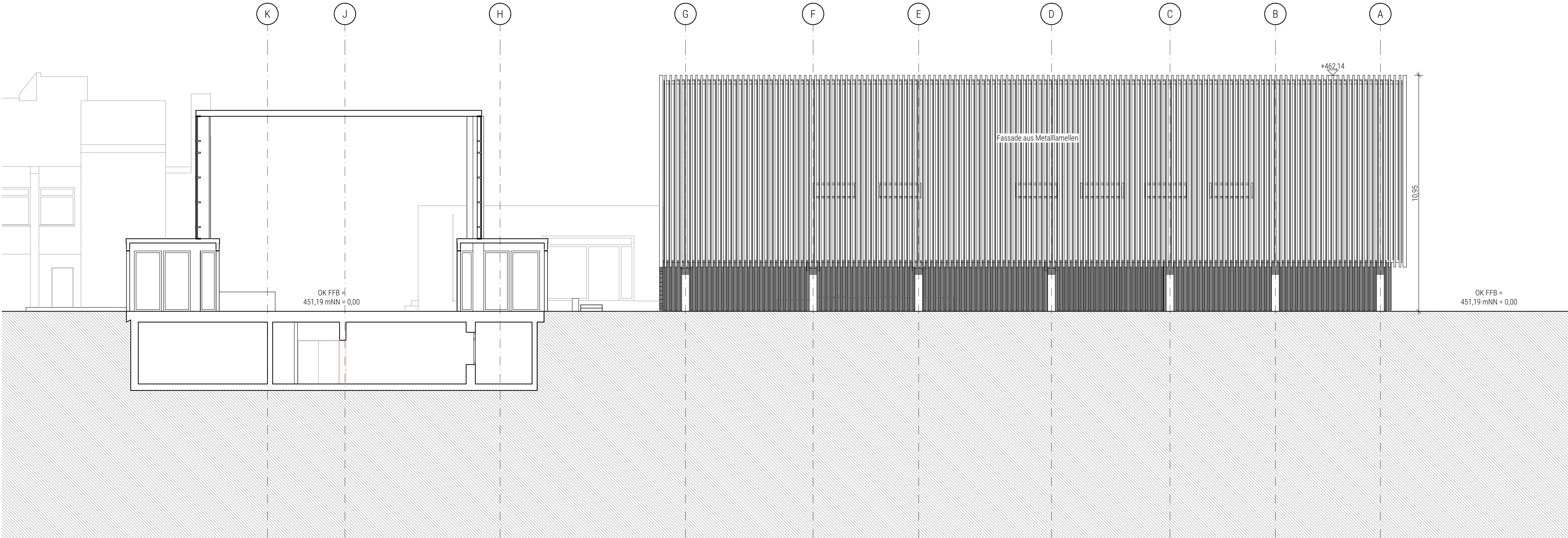
Nordansicht 1:100
