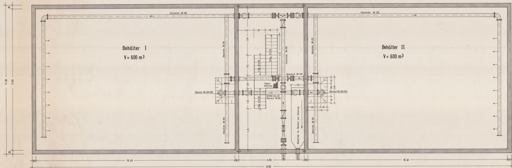
Draufsicht Behälter u. Schieberkammer
