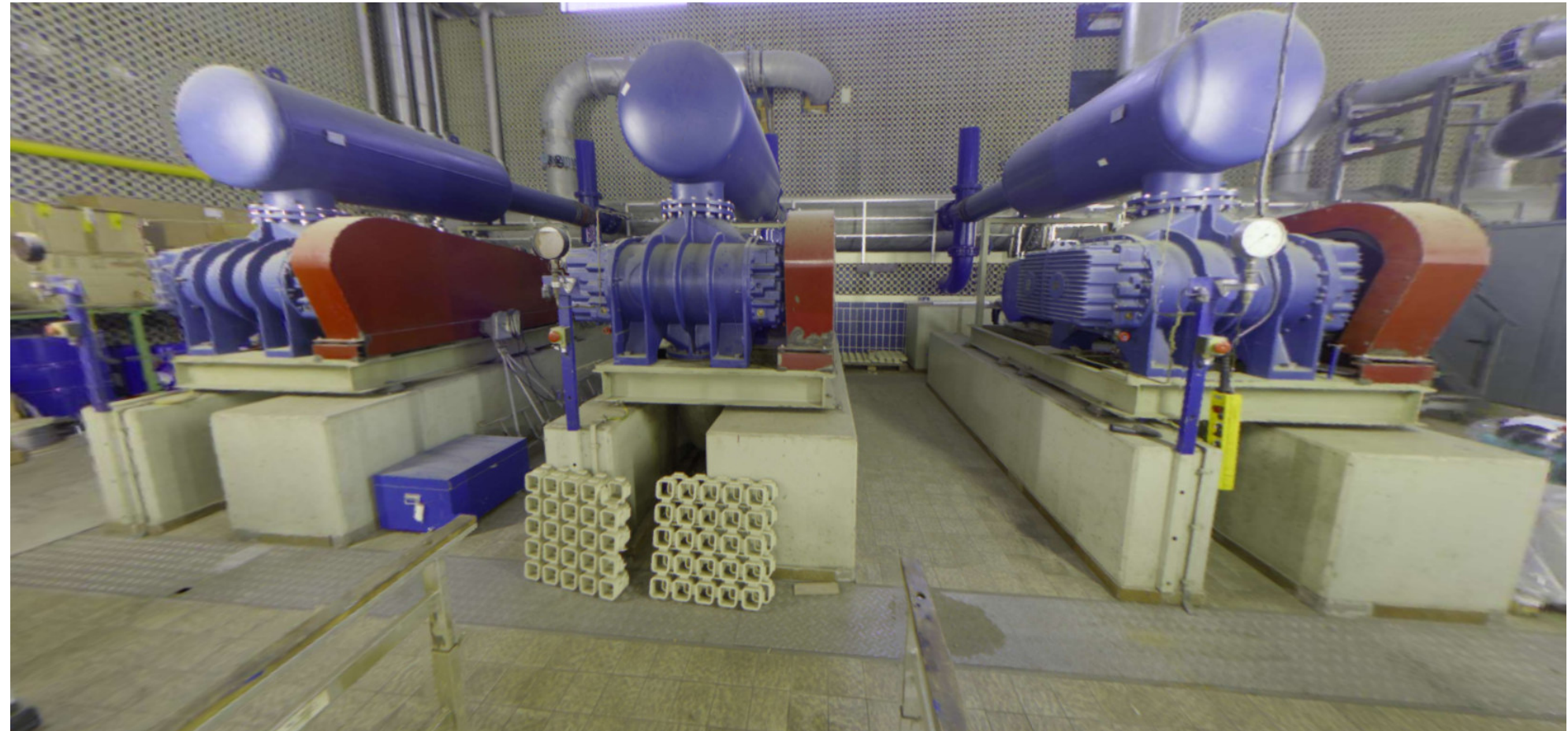
Abbildung 1: Vorderansicht der Fundamente
