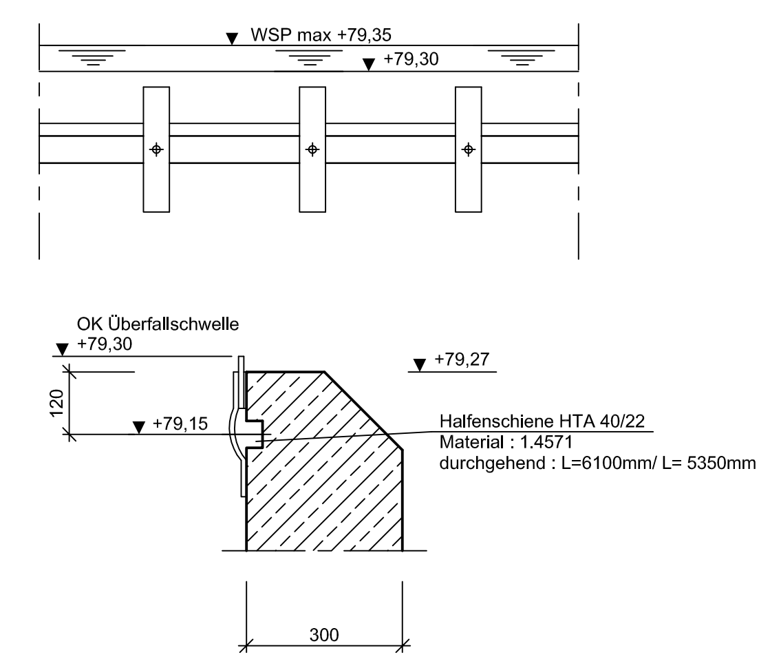
Detail Überfallwehr M. 1:10
