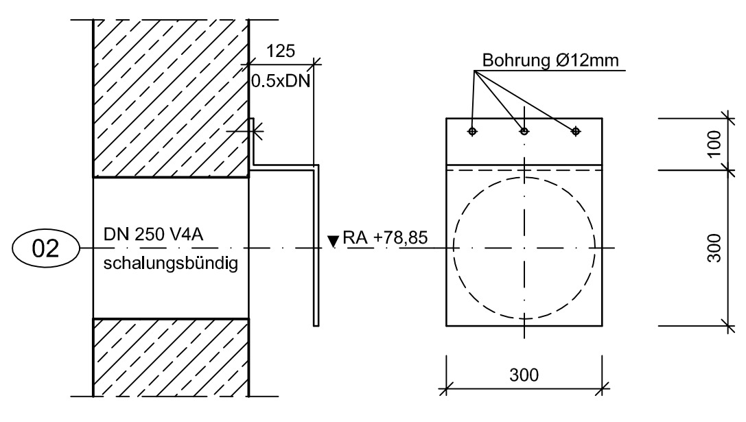
Detail Einlauf Becken mit Prallteller M. 1:10 Anfertigung: 12 SGG
