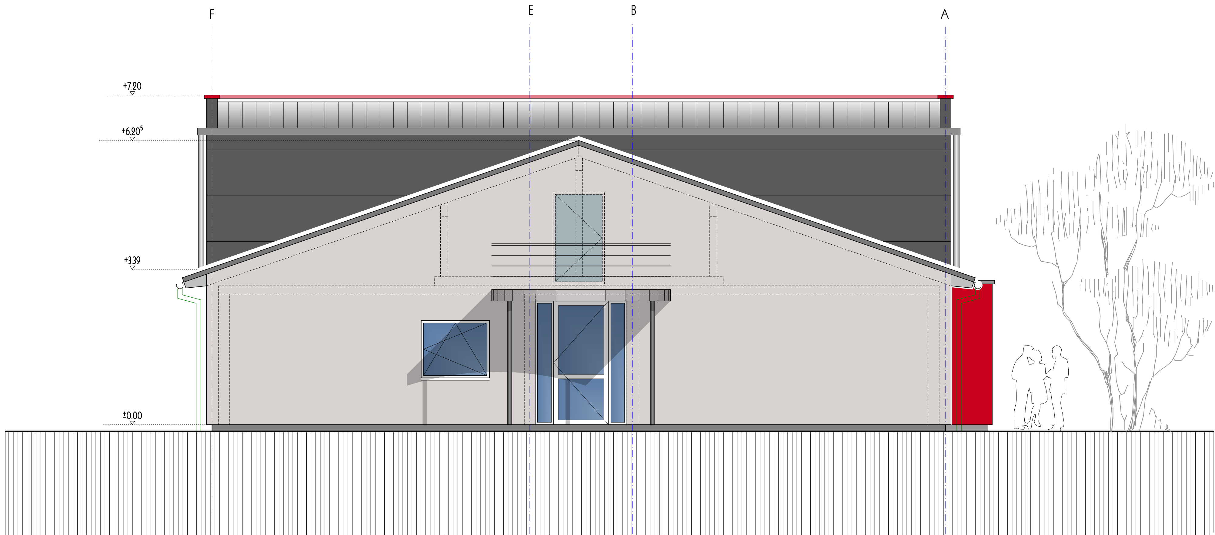
rückansicht
