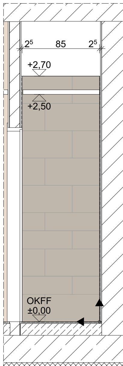
Wandansicht B
