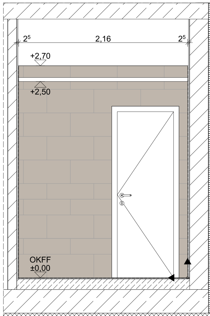
Wandansicht D
