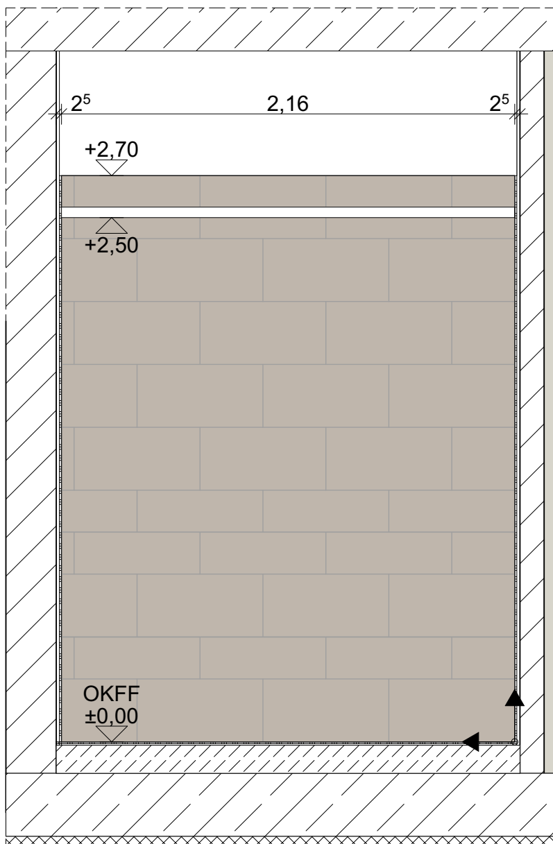
Wandansicht C
