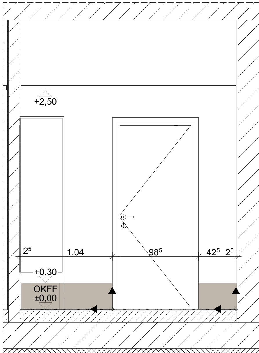
Wandansicht D
