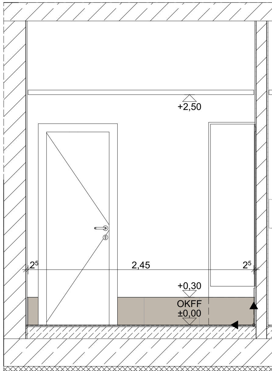
Wandansicht C
