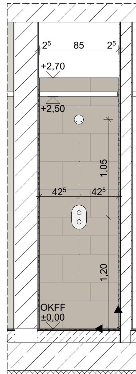
Wandansicht A
