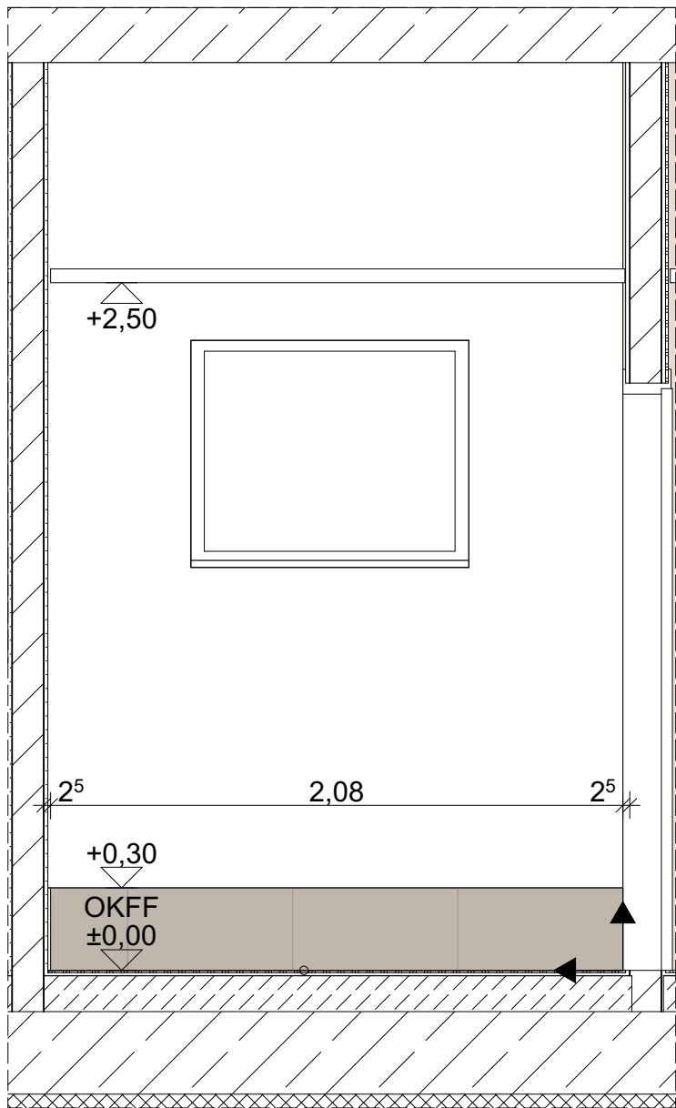
Wandansicht B
