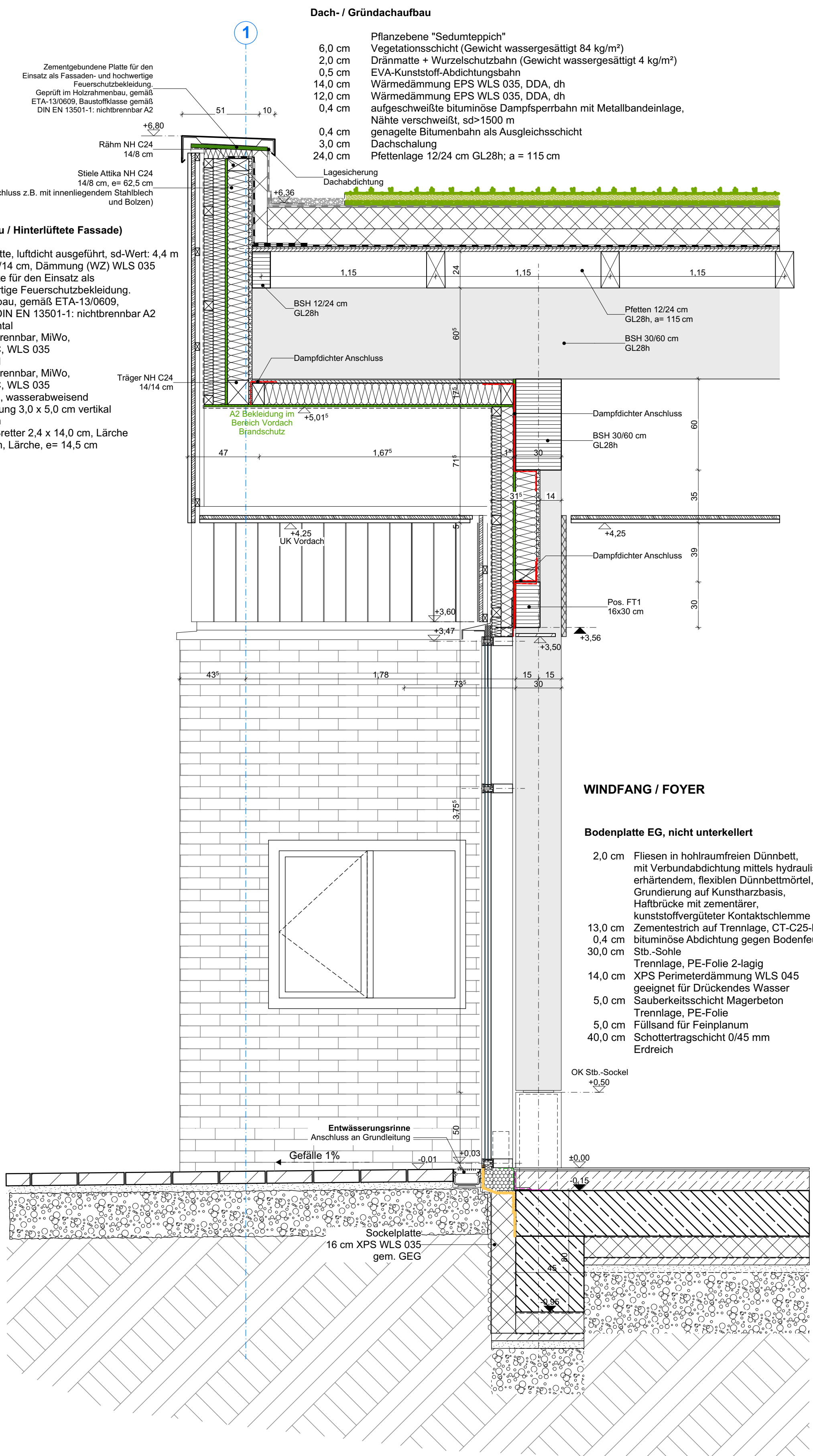
Fassadenschnitt (FAS) 6
