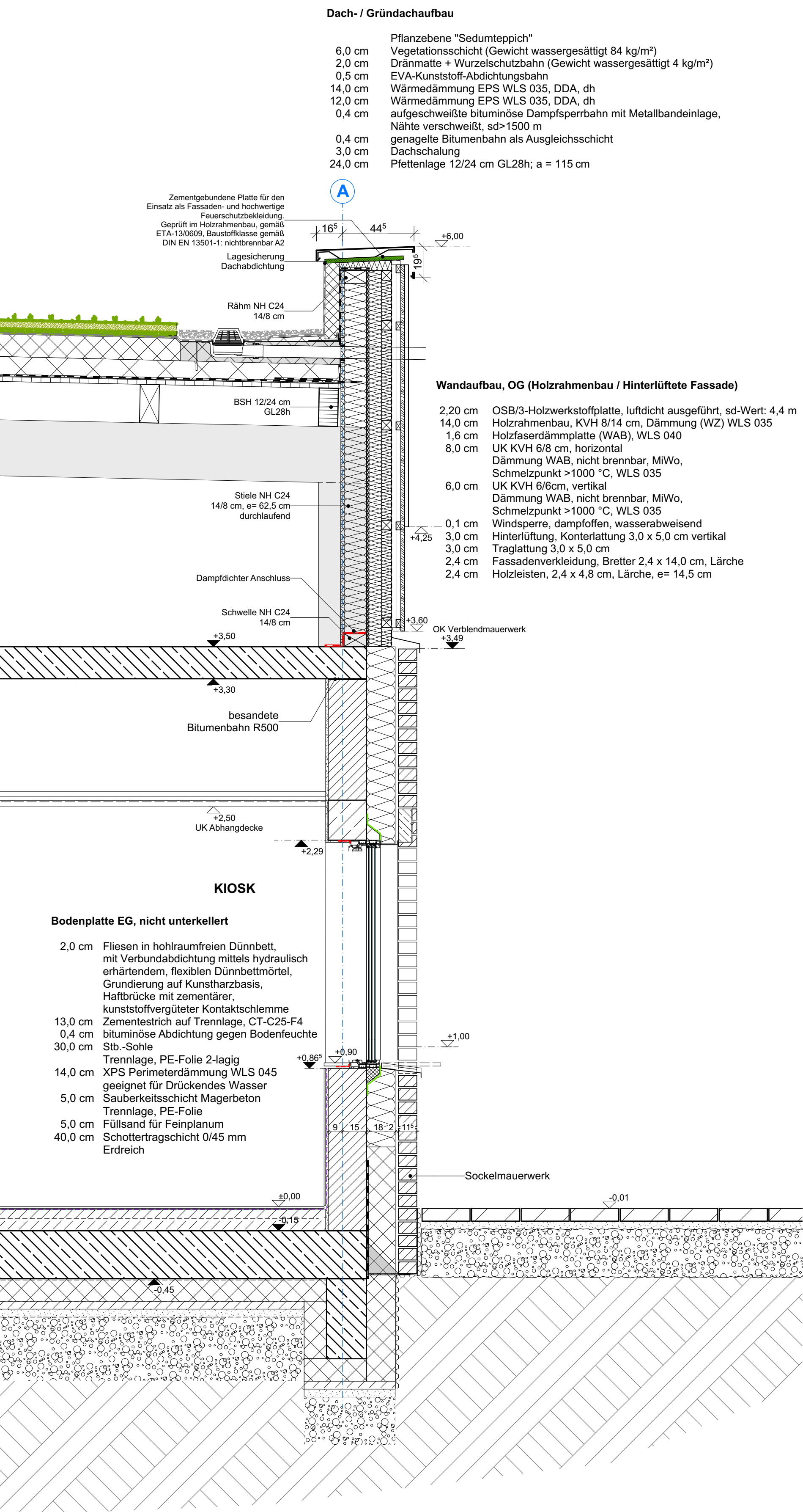
Fassadenschnitt (FAS) 5
