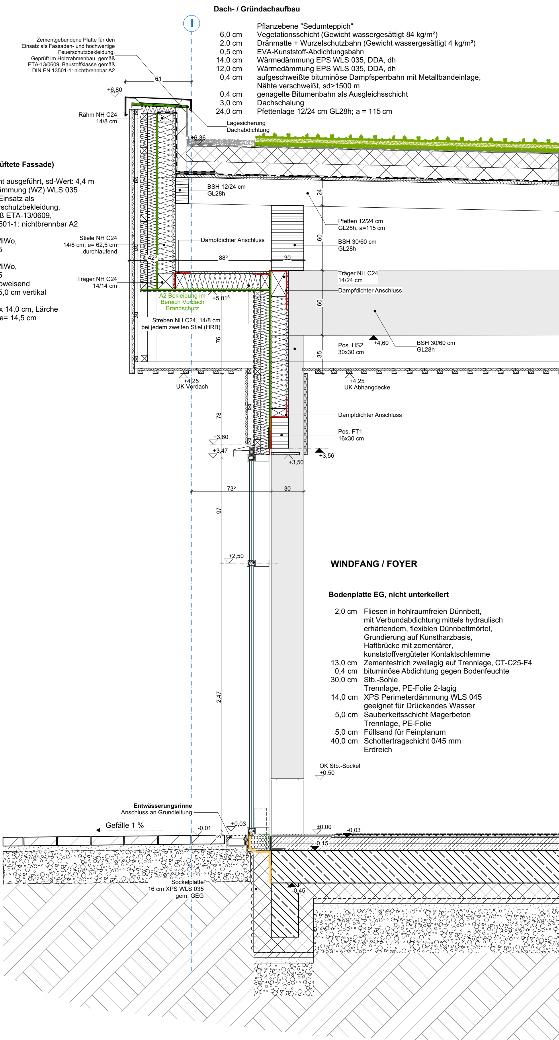
Fassadenschnitt (FAS) 4
