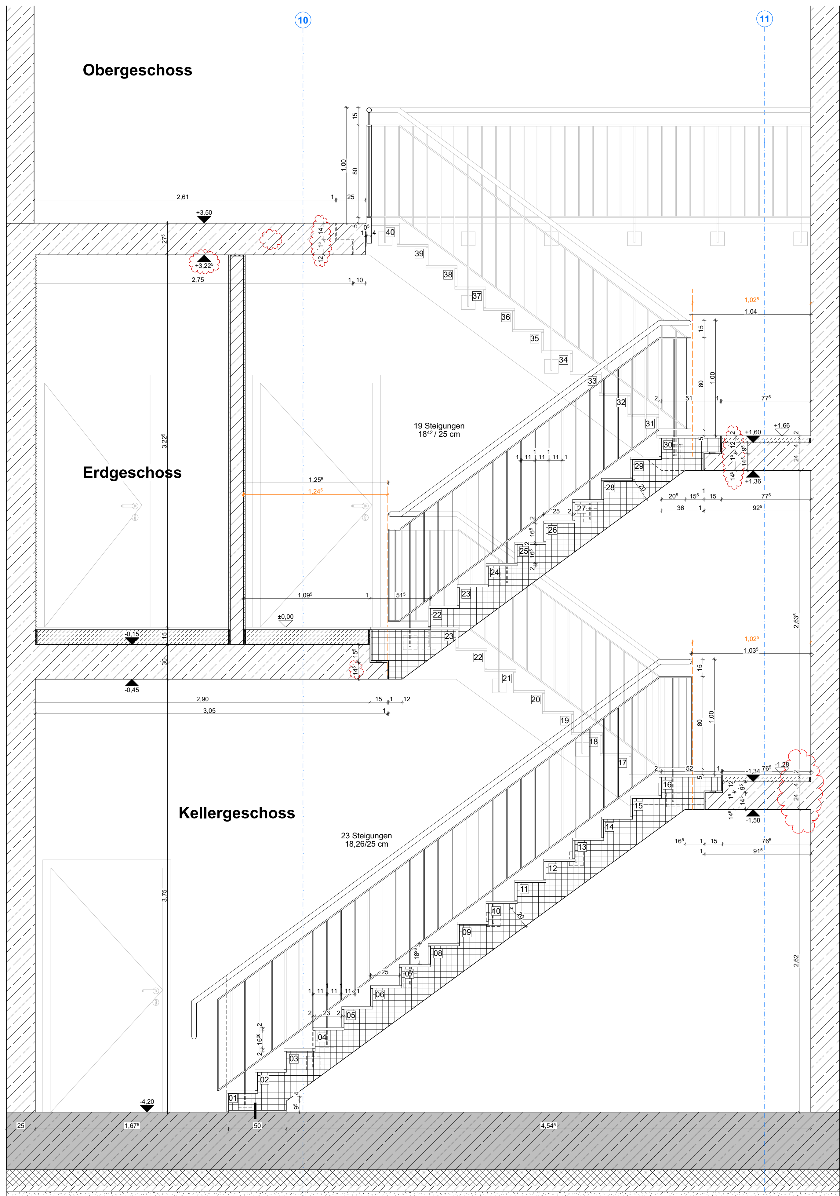
Schnitt 1-1
