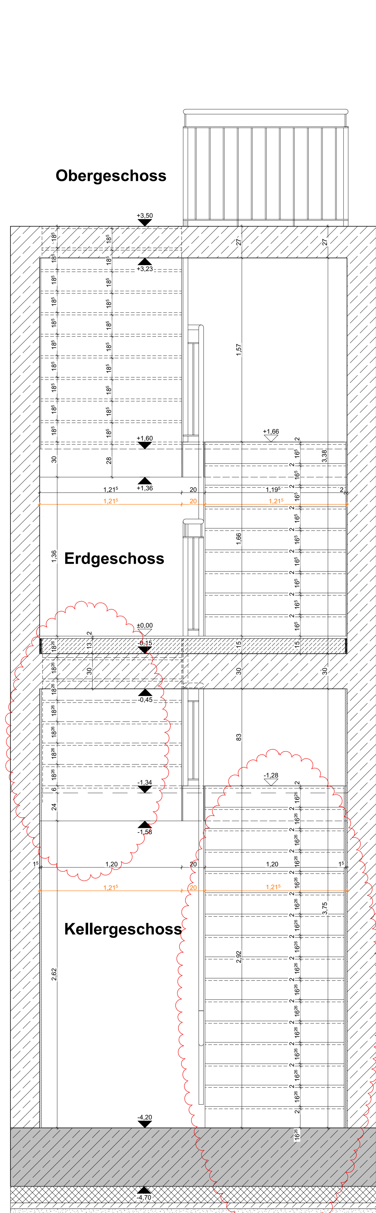
Schnitt 3-3
