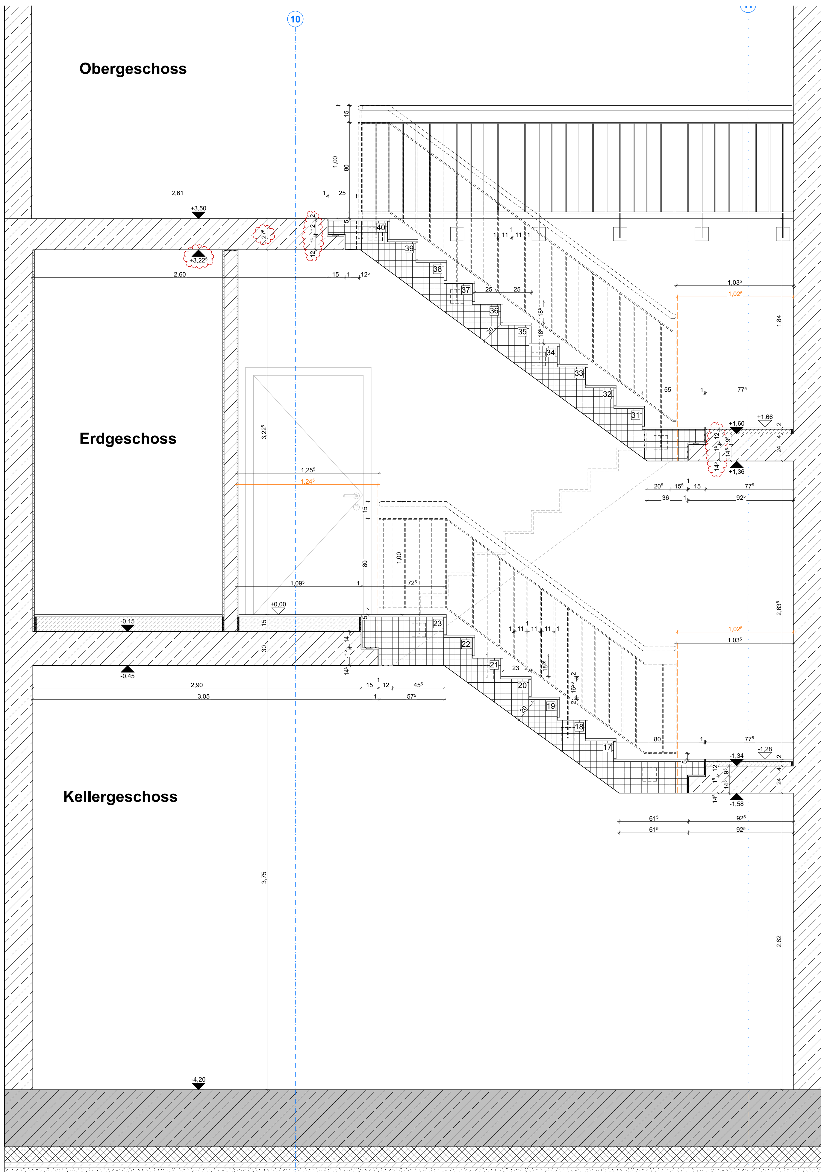
Schnitt 2-2
