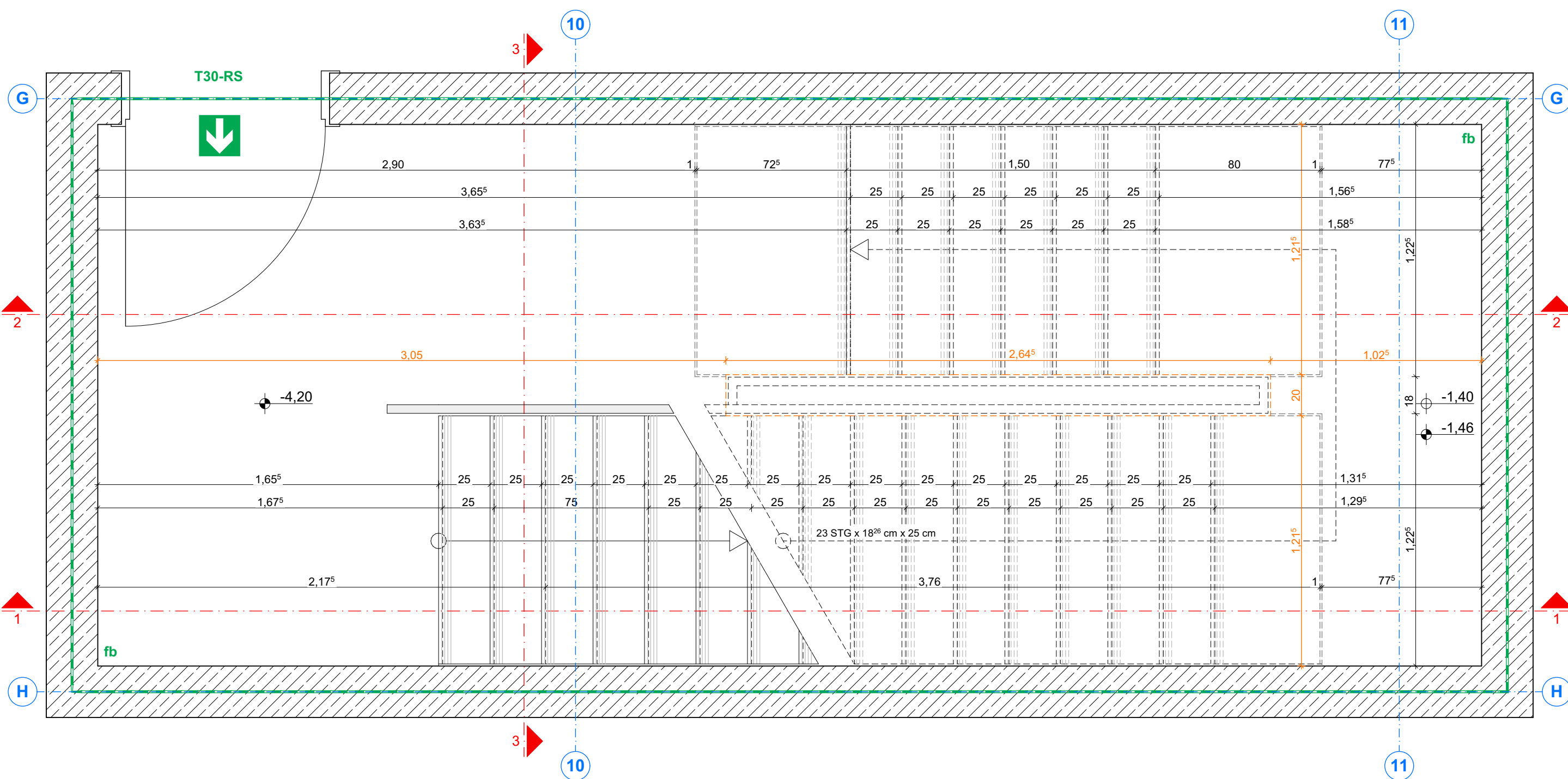
Kellergeschoss
