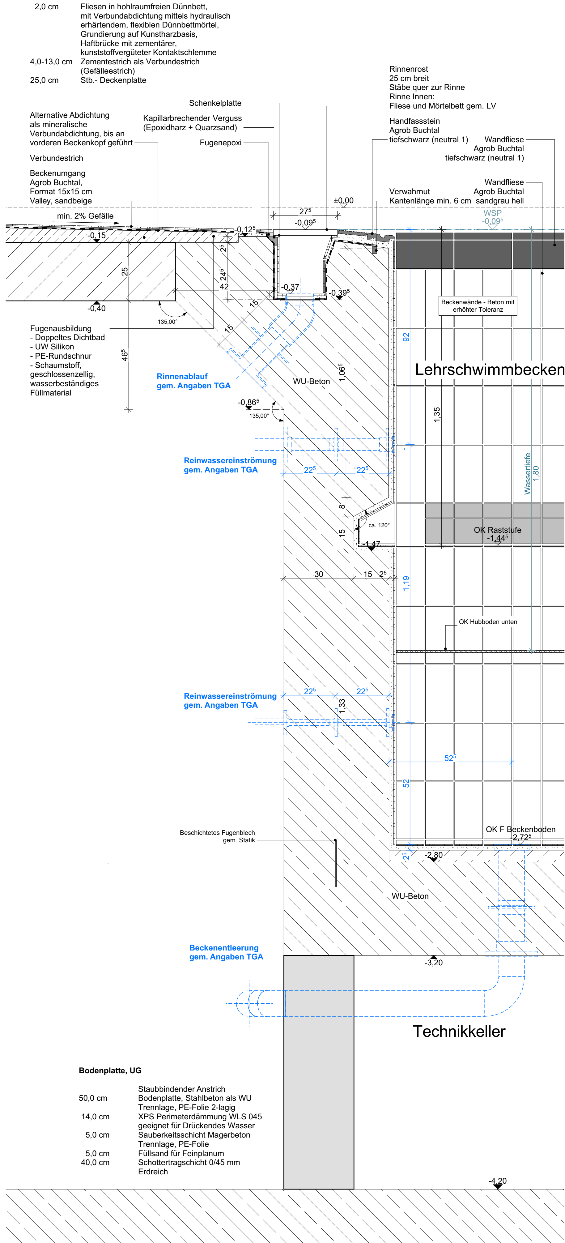
Detail 1:10 Beckenwand / Raststufe
