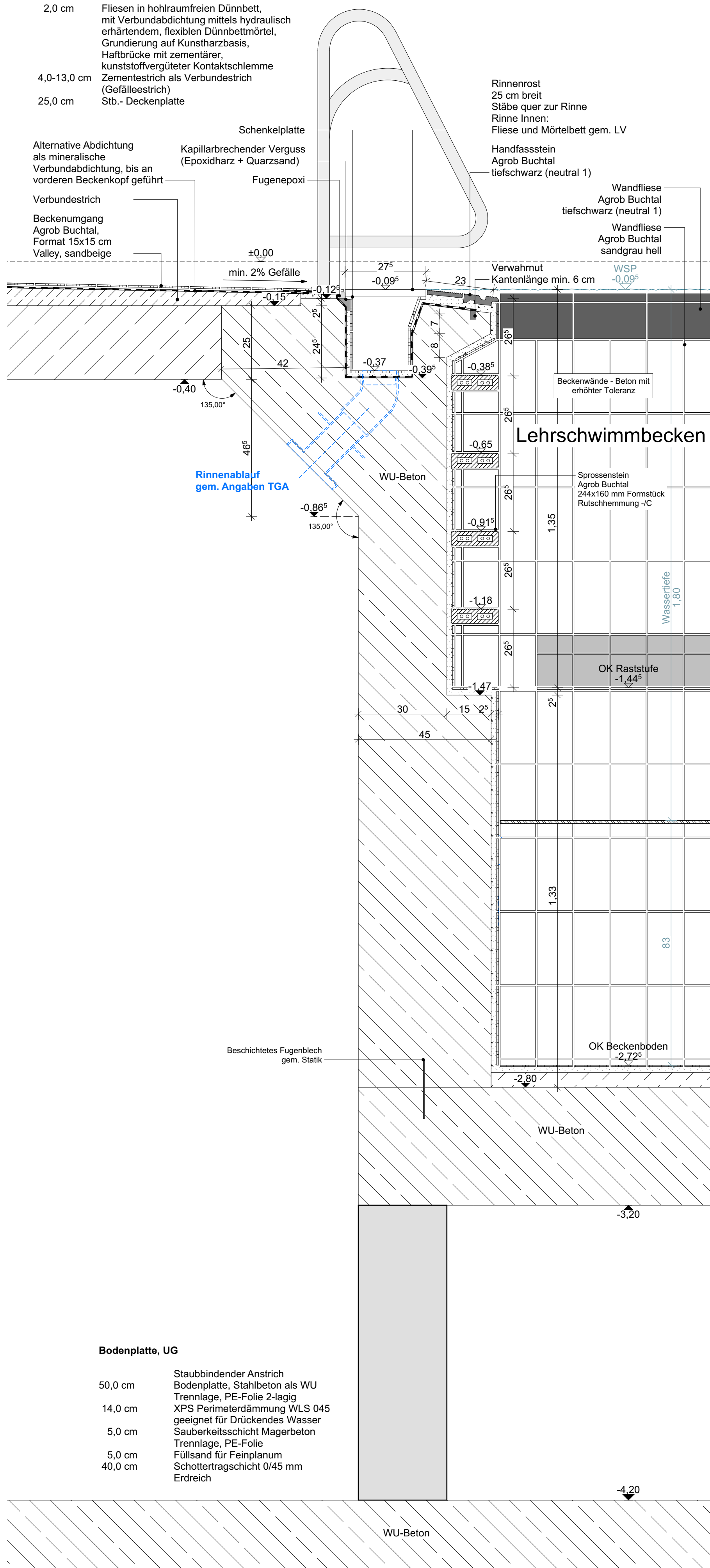
Detail 1:10 Beckenleiter (Schnitt)
