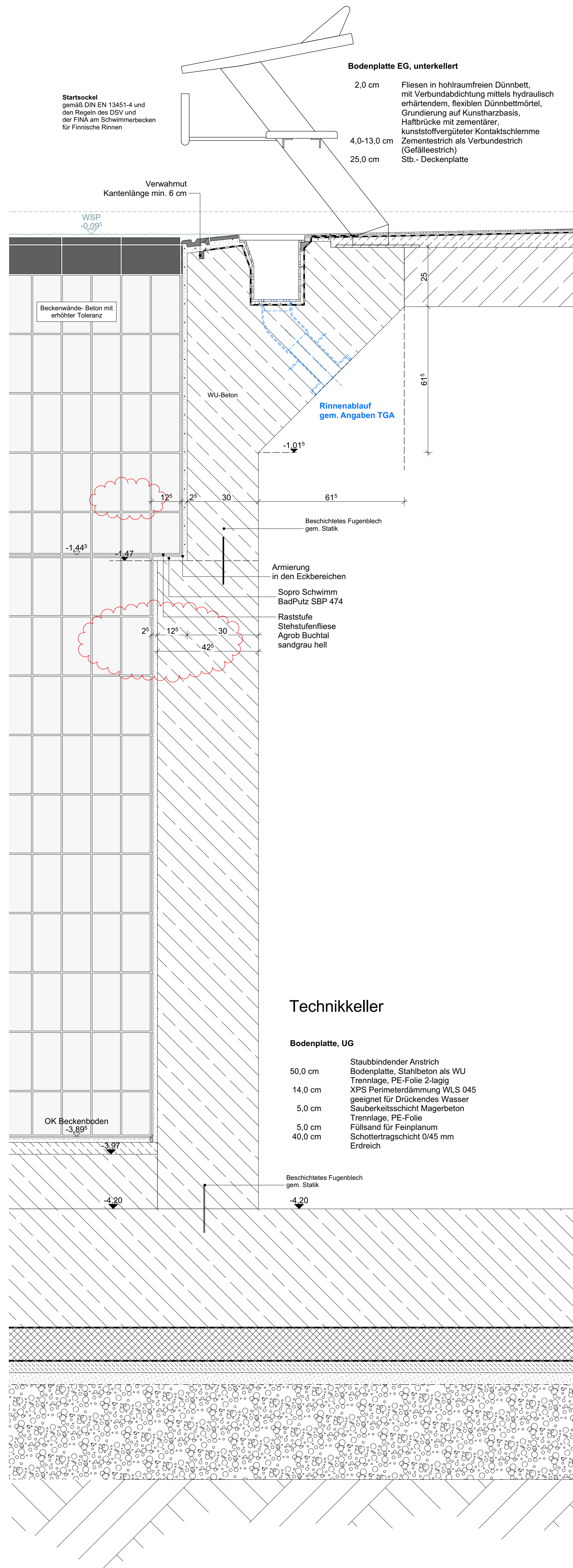
Detail 1:10 Schwimmerbecken WT 3,80 m
