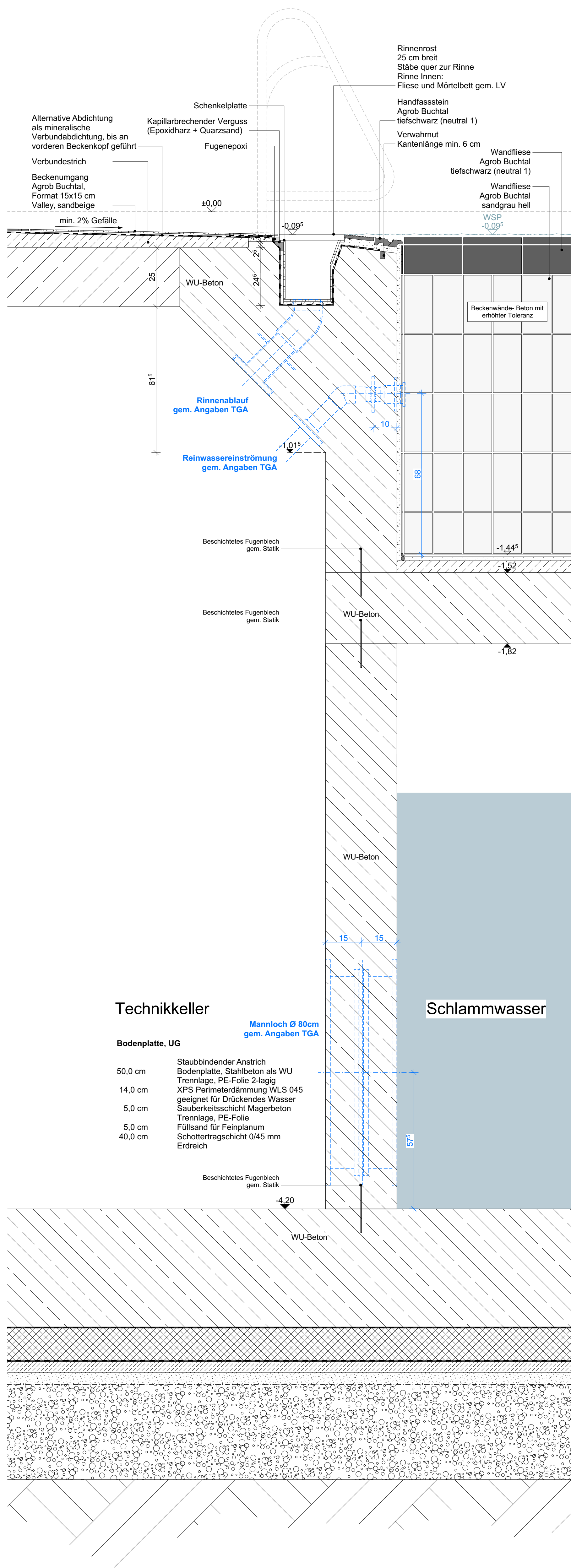
Detail 1:10 Schwimmerbecken WT 1,35 m
