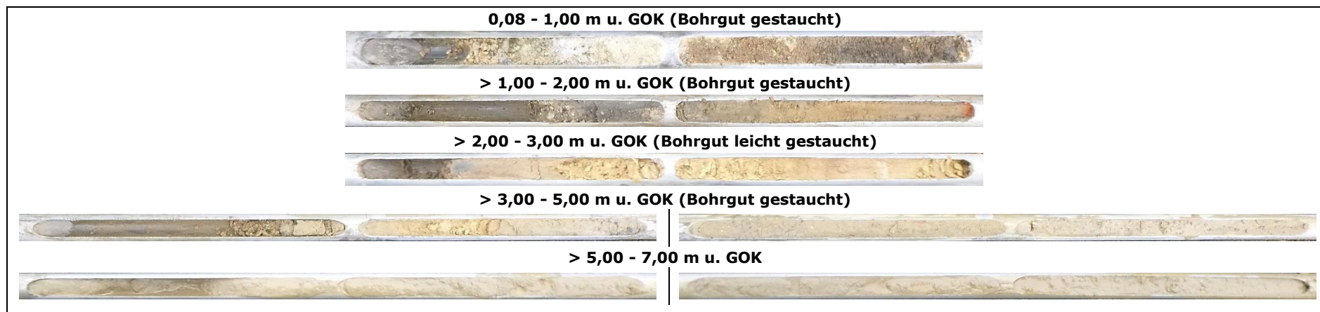
Abb. 18: Bohrgut aus KRB 8
