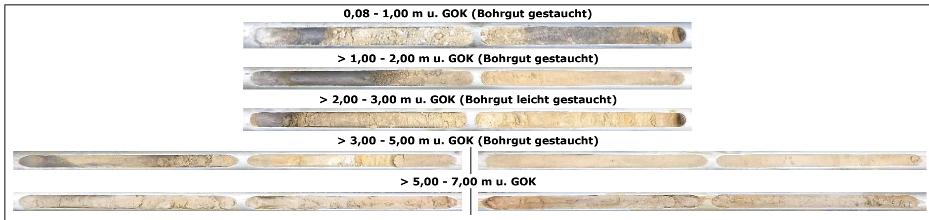
Abb. 14: Bohrgut aus KRB 6
