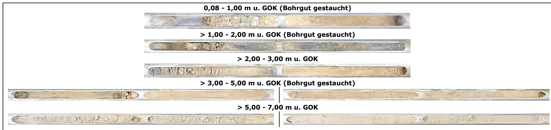
Abb. 9: Bohrgut aus KRB 4
