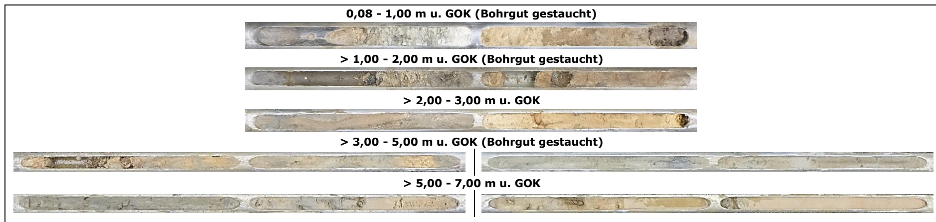
Abb. 7: Bohrngut aus KRB 3
