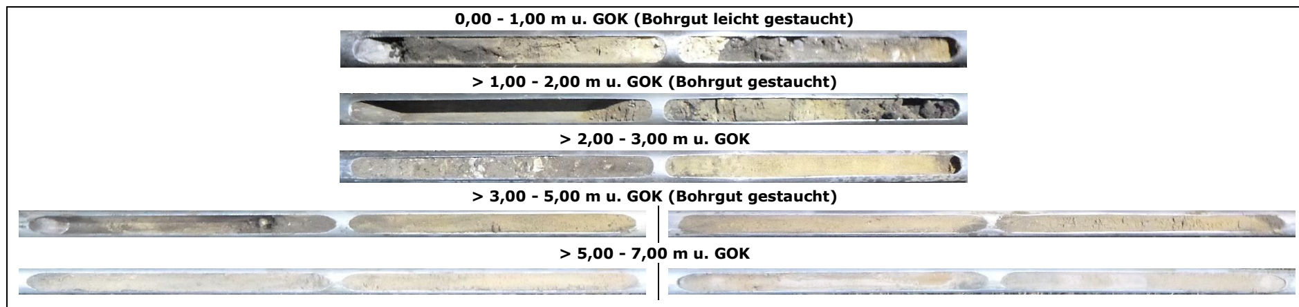
Abb. 16: Bohrgut aus KRB 7
