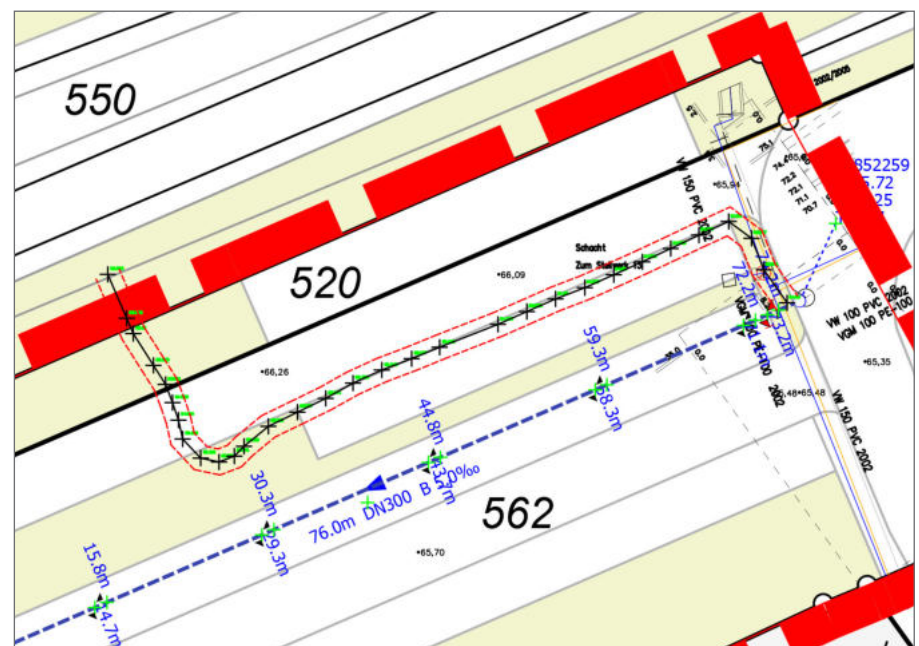
Abb. Vorhandene Leitungstrasse (schwarze Linie, grüne Beschriftung) zzgl. zu berücksichtigende Abstände (rote Strichlinie) (Quelle: Westfalen Weser Netz GmbH 2023)
