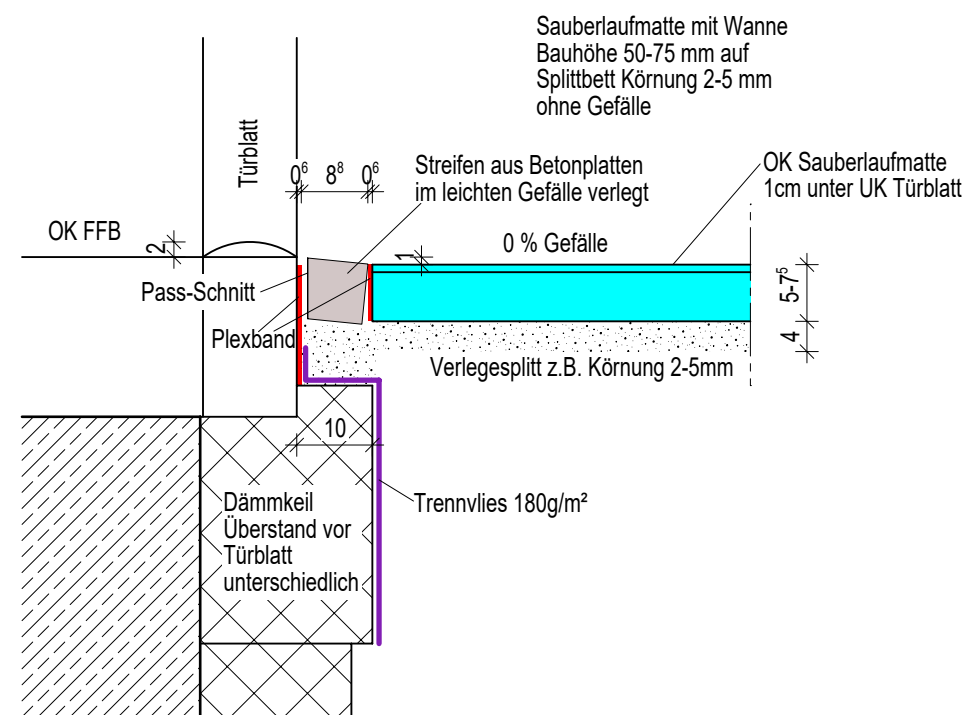
Detail Rost Foyer M 1 : 10
