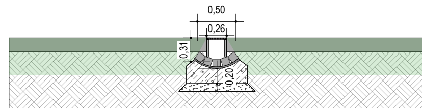
Schnitt 2 - Querschnitt
