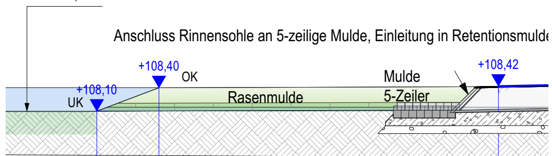
Schnitt 1 - Längsschnitt
